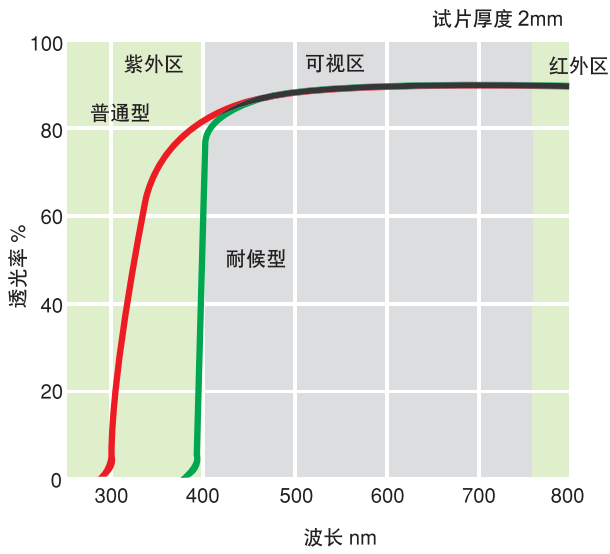
图 22 Panlite 的透光特性
