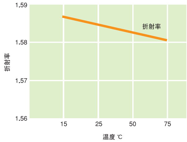
图 23 Panlite 的折射率和温度的关系
