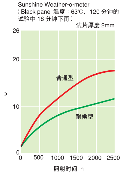
图 30 Panlite 的加速耐候试验 (YI:黄色指数)
