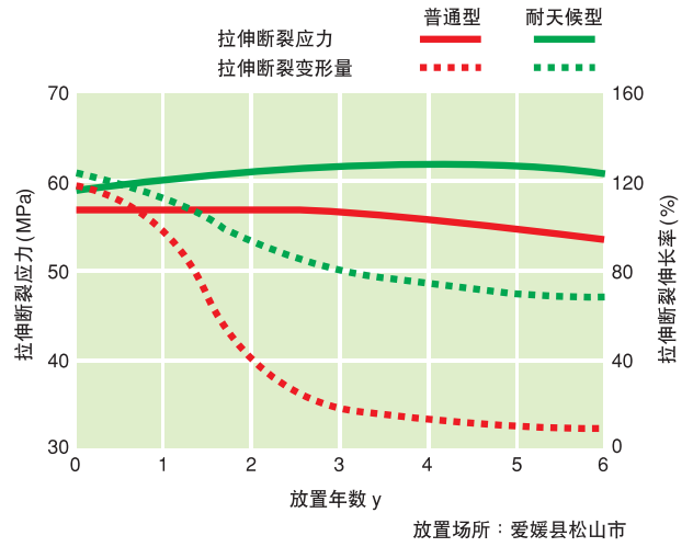
图 24 Panlite 的室外放置试验(拉伸特性)
