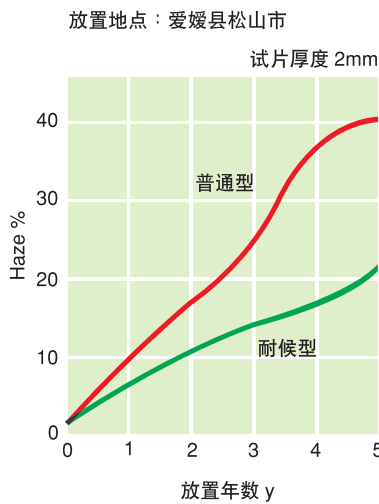
图 26 Panlite 的室外放置试验 (Haze:雾度)
