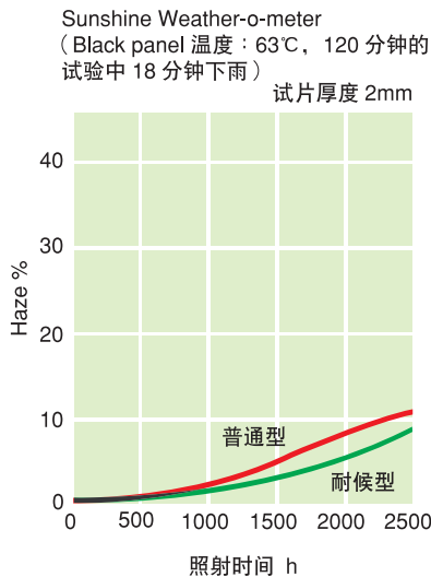
图 29 Panlite 的加速耐候试验 (Haze:雾度)
