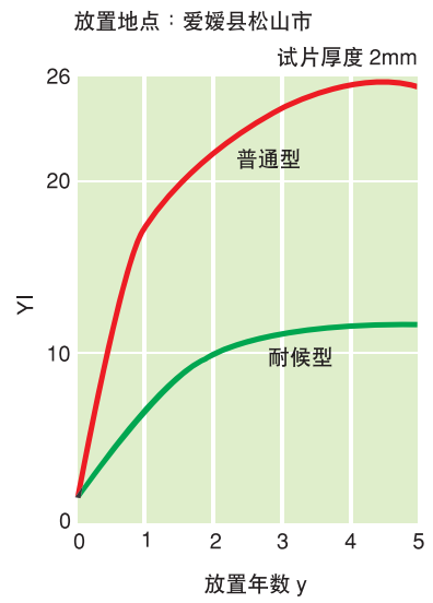
图 27 Panlite 的室外放置试验 (YI:黄色指数)
