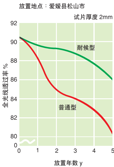
图 25 Panlite 的室外放置试验 (全光线透过率)
