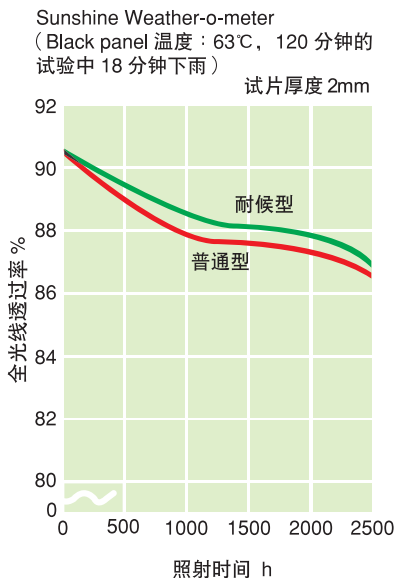
图 28 Panlite 的加速耐候试验 (全光线透过率)
