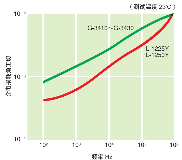
图19 Panlite 在不同频率时的介电损耗角正切
