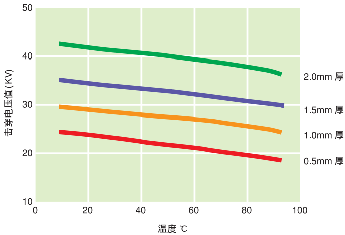
图14 Panlite 在不同温度条件下的绝缘破坏电压
