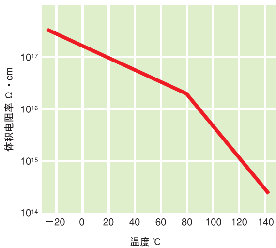
图15 Panlite 在不同温度条件下的体积电阻率
