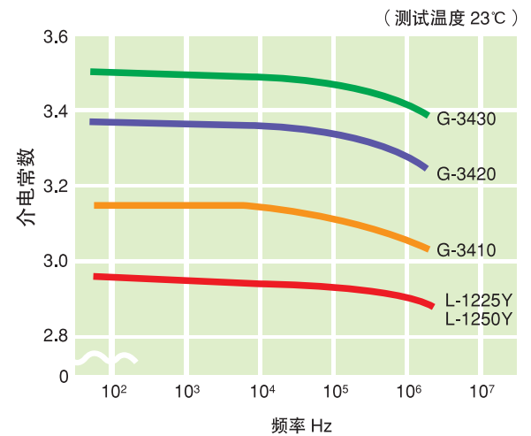
图18 Panlite 在不同频率时的介电常数
