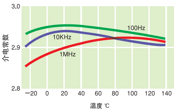
图16 Panlite 的介电率与温度的关系
