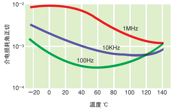
图17 Panlite 的介电损耗角正切与温度的关系
